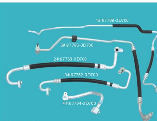
JN-6H001 现代索纳塔 老款管路总成 Hyundai Sonata (old) pipeline assembly
