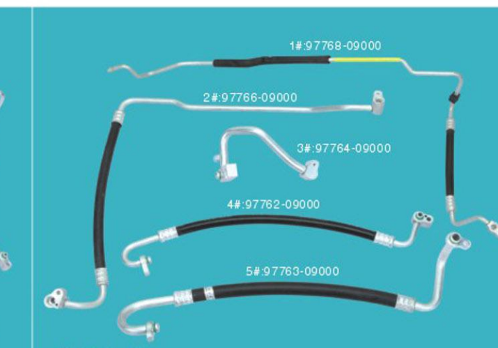
JN-6H002 现代索纳塔 新款管路总成 Hyundai Sonata (new) pipeline assembly
