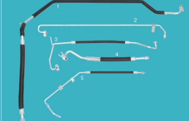
JN-6K004 豪沃 A7 管路总成 Howo A7 pipeline assembly
