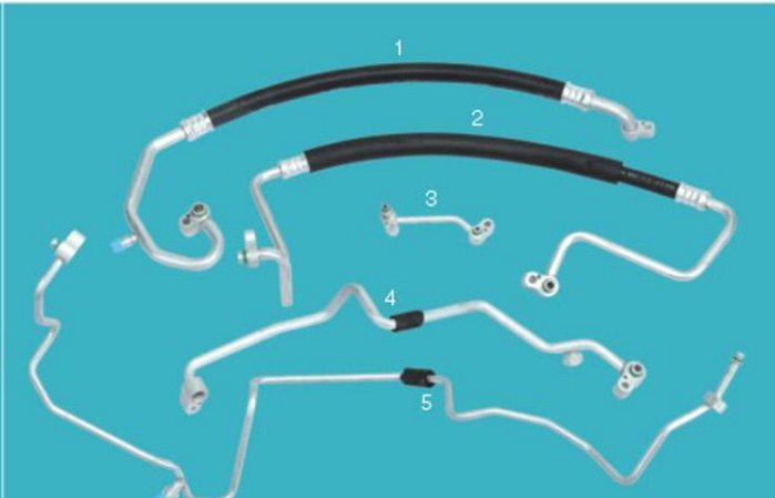
JN-6H020 起亚千里马1.3管路总成 Kia Qianlima 1.3 pipeline assembly
