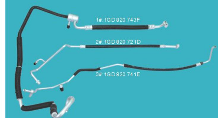
JN-6D017 捷达王 04款管路总成 JETTA GT 04 pipeline assembly
