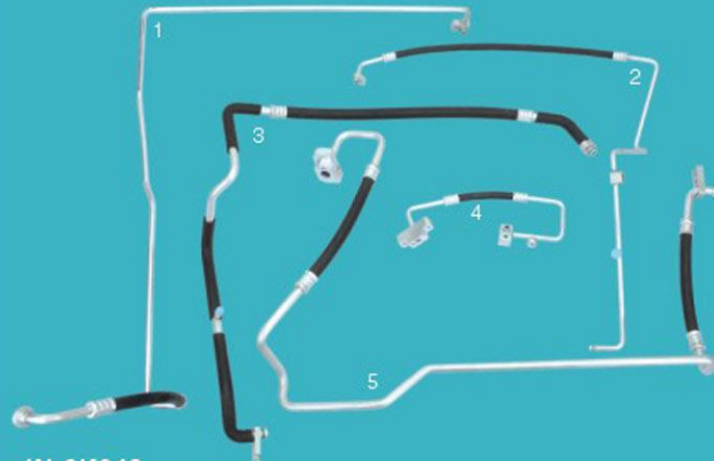
JN-6K018 新大威 10款管路总成 New Dawei 10 pipeline assembly
