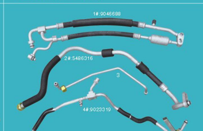
JN-6M004 别克凯越管路总成 Buick Excelle pipeline assembly
